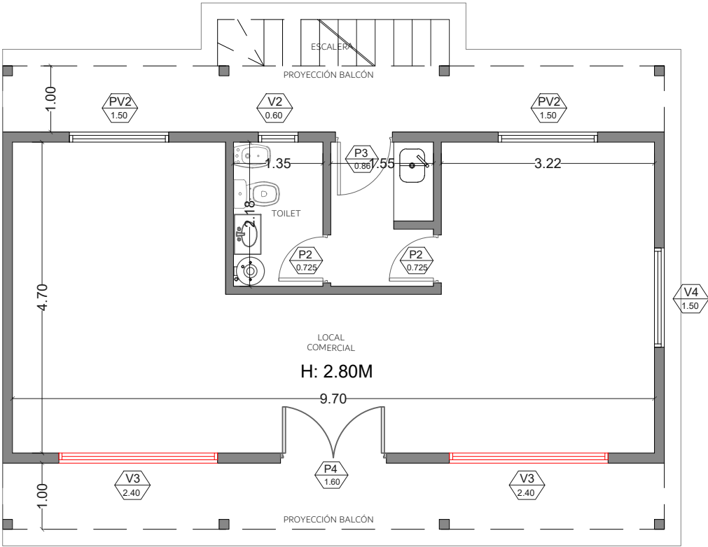
PLANTA BAJA
