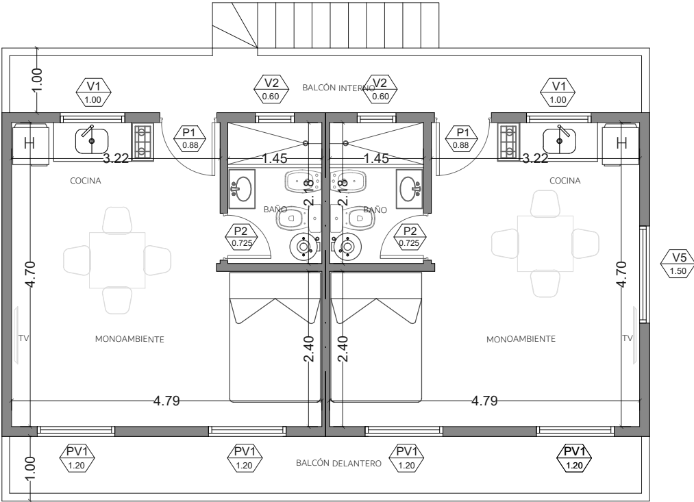
PLANTA ALTA
